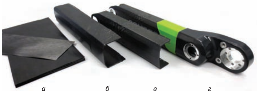
Фото 4. Процесс изготовления руки робота ENGEL e-pic из однонаправленных препрегов состоит из следующих основных технологических операций: а – раскрой однонаправленных препрегов на отдельные слои заданных размеров и сборка из них многослойного пакета-заготовки; б – нагрев пакета-заготовки, его формование и фиксация формы при охлаждении; в – механическая обработка (обрезка кромок, формование отверстия); г – сборка частей изделия между собой и с алюминиевым элементом путем склеивания
