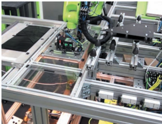
Фото 5. Интегрированная в производственную ячейку видеооптическая система, предназначенная для определения фактического положения слоя однонаправленного препрега на выкладочной головке
