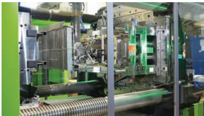
Фото 4. ИК-излучатель с несколькими зонами нагрева пленки интегрирован в захват линейного робота
