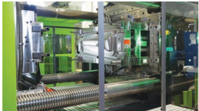
Фото 3. Литьевая форма, в которой в процессе текстурирования по методу In-Mould Graining пленка приобретает требуемую поверхностную структуру
